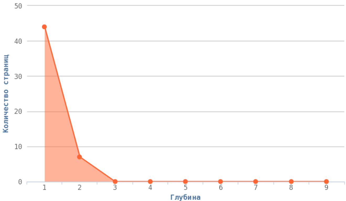
Глубины страниц
